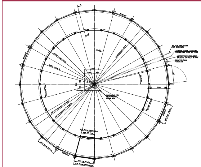
Führanlage mit Hufschlagdach, Typ Eco, Grundriss
